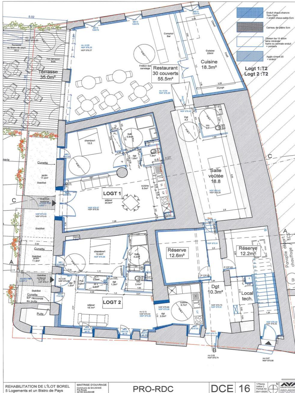
Plan du RDC comprenant la terrasse, le restaurant, la cuisine, la salle voûtée et les deux réserves
